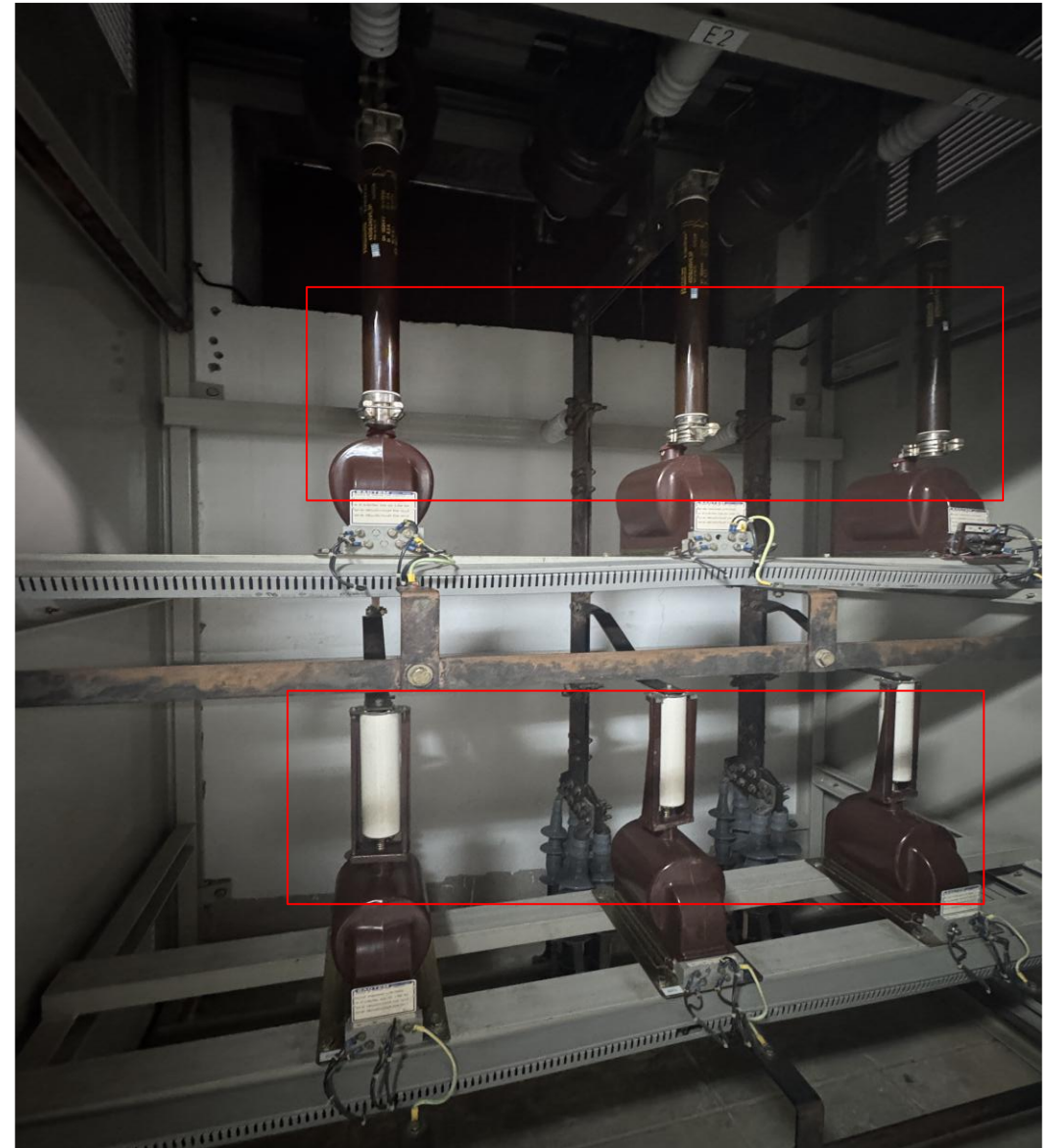
V.5 - Các TU đo áp
