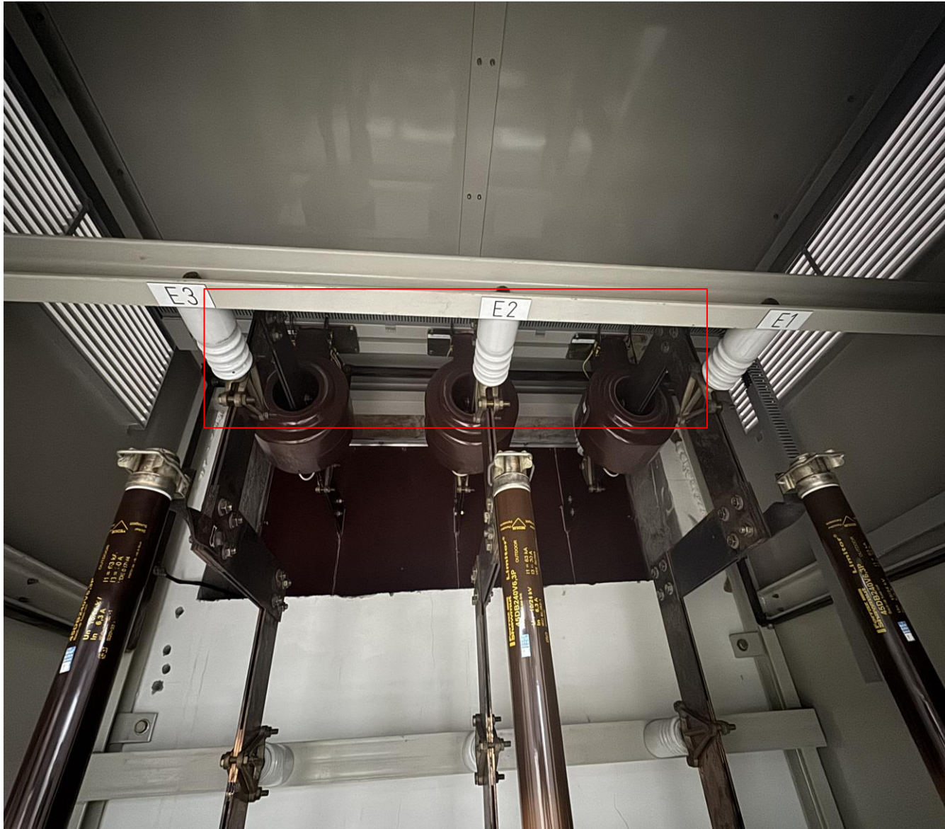
V.4 - Các TI đo dòng
