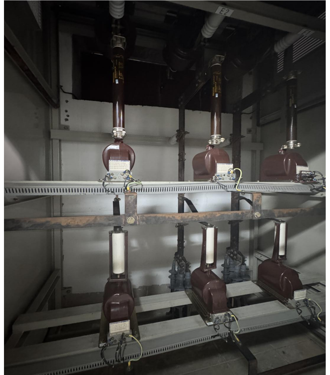
V.1 – Tủ đầu ra máy phát 01GTA021AR
